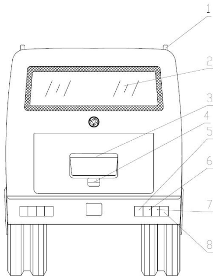
EQ6680ZT6D 后围图（挡风玻璃结构）
